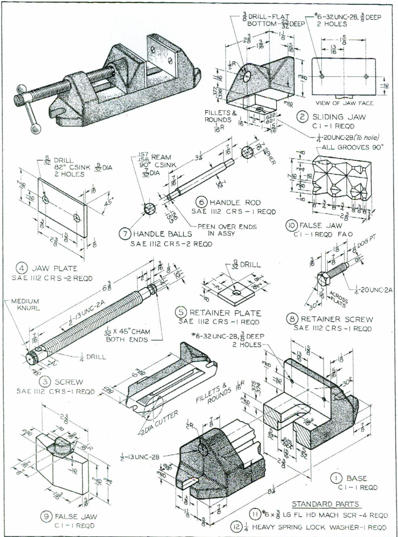
Fig. 16-44. Drill press vise.
